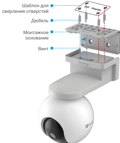
Рисунок 1. Монтаж на потолок
