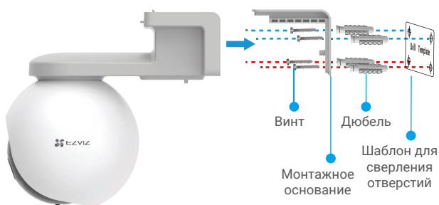
Рисунок 2. Монтаж на стену
